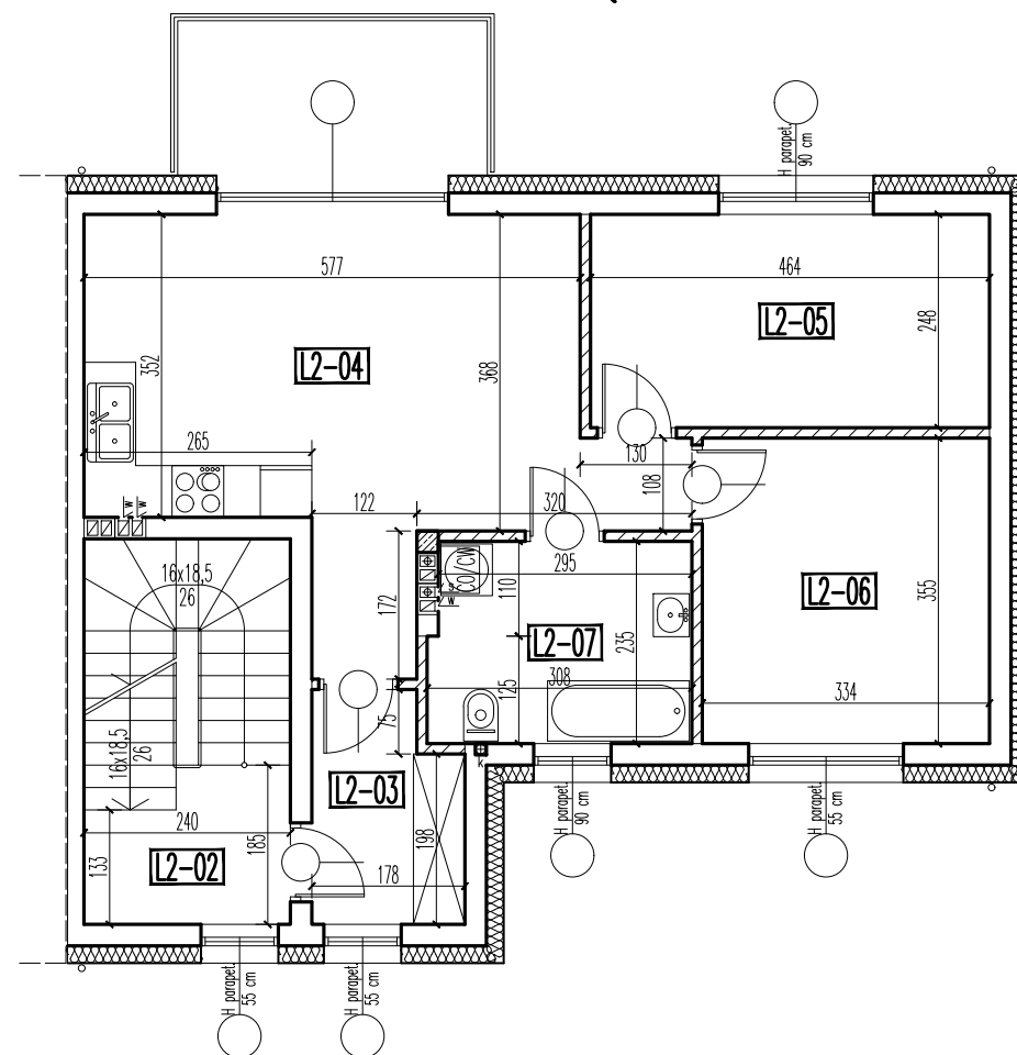
RZUT PIĘTRA
